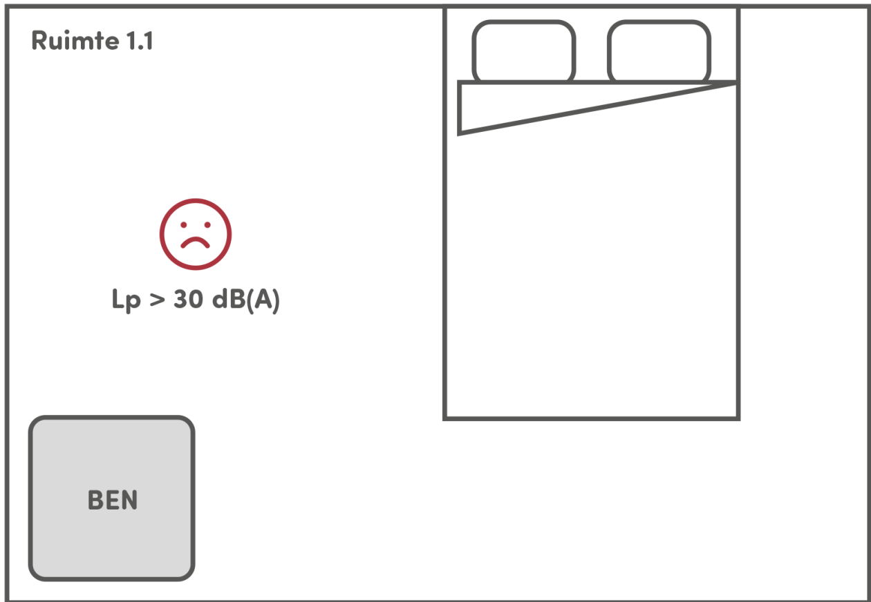
Figuur 2: Schets van de situatie in Voorbeeld 1. De BEN Dual-AIR warmtepomp staat in de hoek van een slaapkamer (ruimte 1.1). Het geluiddrukkniveau ( L_p ) komt boven de 30 dB(A) uit. In het geval dat dit een verblijfruimte is, kan de het apparaat hier niet geplaatst worden.
