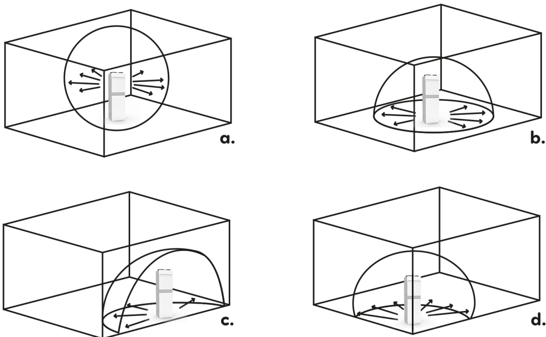
Figuur 5: Verspreiding van geluid vanaf de geluidsbron op verschillende posities in de ruimte. Met in (a) de geluidsbron in de vrije ruimte, (b) op de grond, (c) op de grond bij een muur en (d) op de grond in een hoek. Het geluid spreidt zich respectievelijk uit over een hele, een halve, een vierde en een achtste bol.
