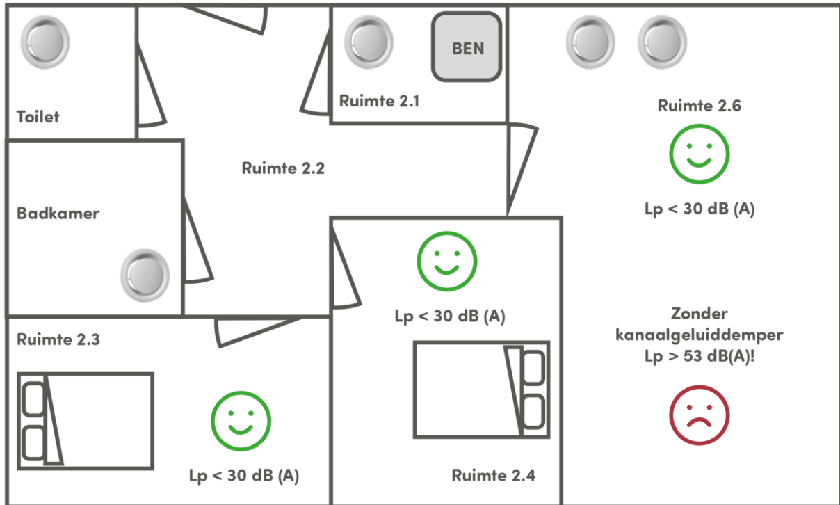
Figuur 3: Schets van de situatie in Voorbeeld 2. De BEN Dual-AIR warmtepomp staat in een systeemruimte van een appartement (ruimte 2.1). Het geluidrukniveau ( L_p ) in de slaapkamers (Ruimte 2.3 en 2.4) blijft ver onder de 30 dB(A).
