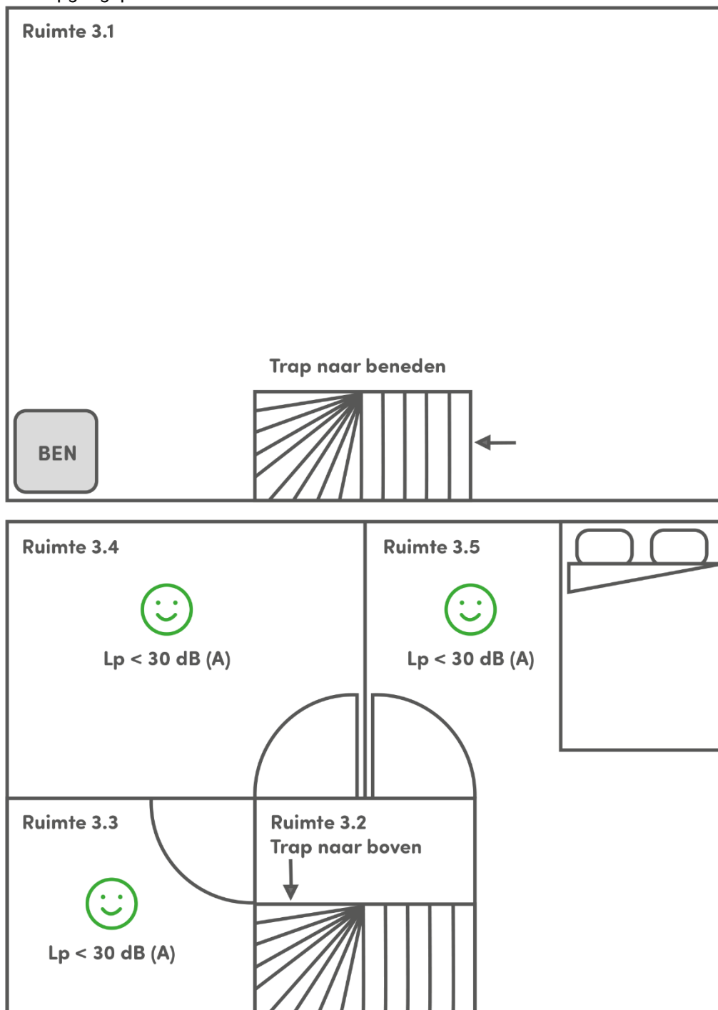
Figuur 4: Schets van de situatie in Voorbeeld 3. In het bovenste plaatje: de open zolder met een open trapgat naar beneden en met de BEN Dual-AIR in een van de hoeken. In het onderste plaatje: de verdieping onder de zolder met een overloop (ruimte 3.2) onderaan de trap naar de zolder en drie ruimtes (ruimte 3.3; 3.4 en 3.5). Deze drie ruimtes hebben ieder een wand met een deur naar de overloop.
